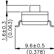
EXTENDED ACTUATOR
