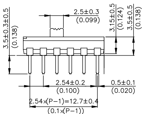
EXTENDED ACTUATOR
