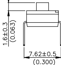
EXTENDED ACTUATOR
